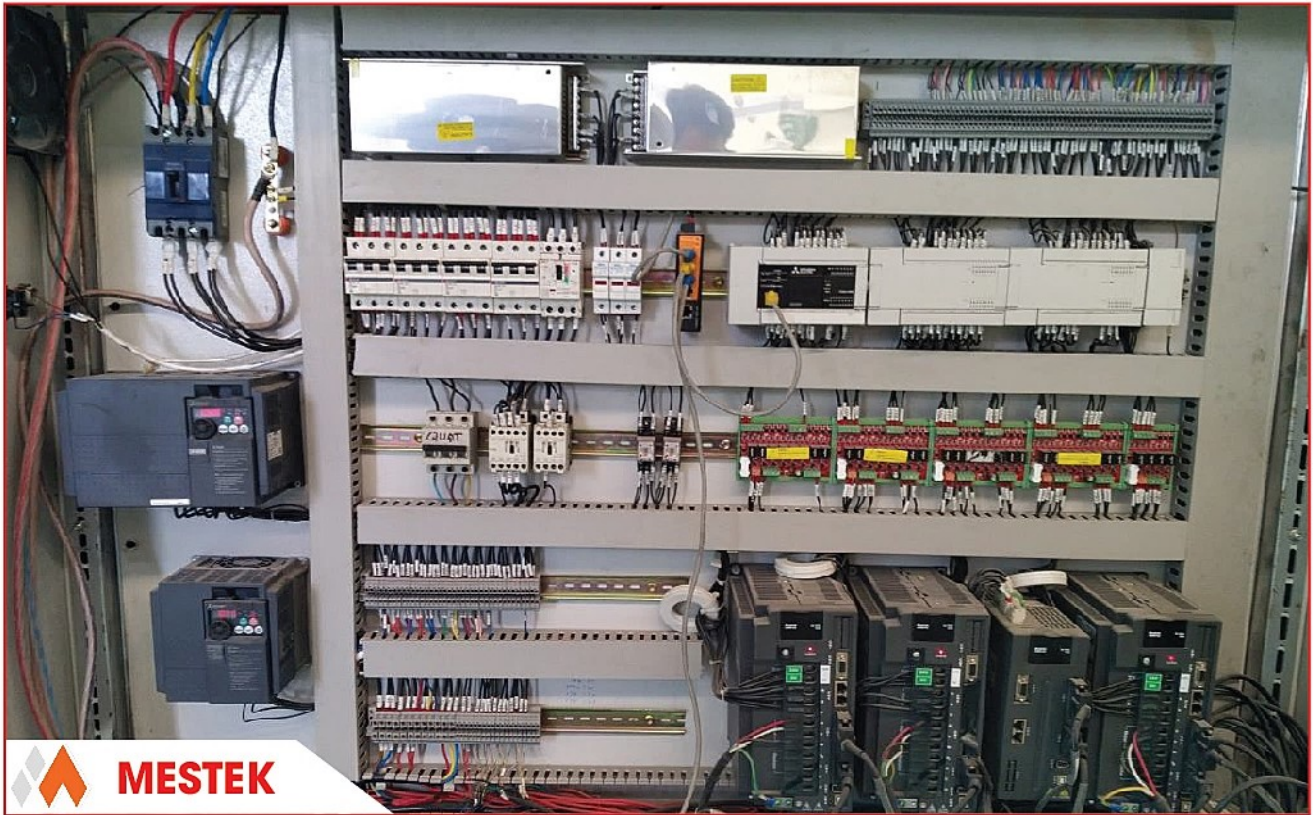
Tủ điều máy hàn giàn giáo tự động Công ty TNHH Daiichi Group – Thanh Xuân, Hà Nội
