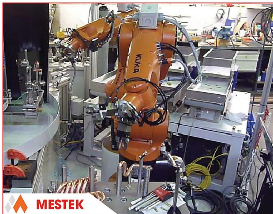
Thiết kế, chế tạo và lắp đặt dây chuyền robot hàn ống Công Ty Ô tô Toyota Việt Nam - Phúc Thắng, Phúc Yên, Vĩnh Phúc
