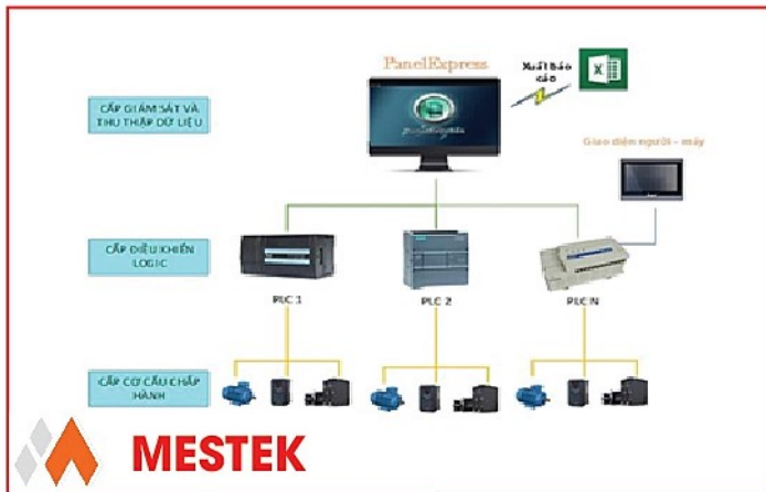
Hệ thống giám sát thiết bị nhà máy
