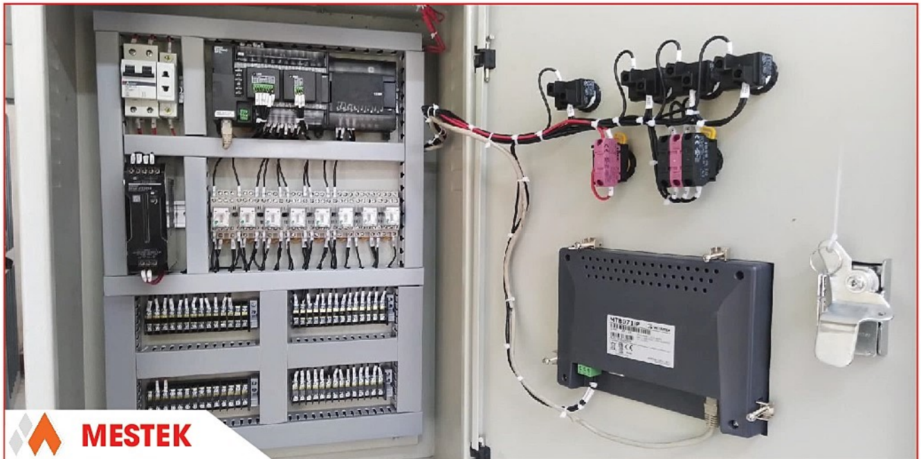
Dự án Lắp đặt tủ điều khiển hệ thống HVAC
