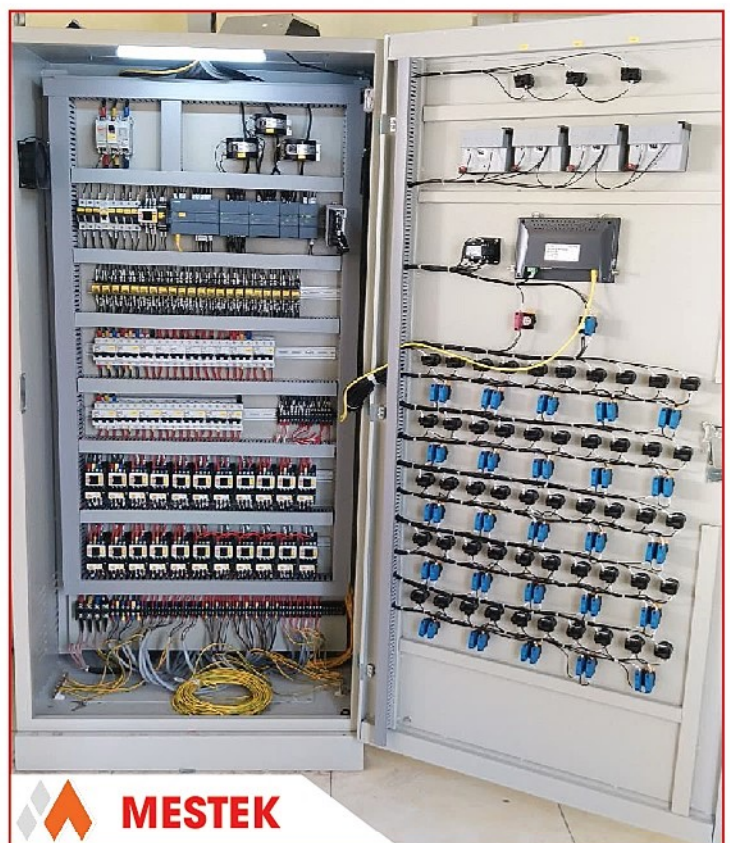
Tủ điều khiển hệ thống transerver lắp ráp ô tô
