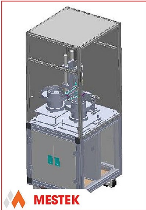
Thiết kế, chế tạo và lắp đặt máy rửa hóa chất tự động Công Ty TNHH Ogino Việt Nam - KCN Vsip, Phù Chấn, Từ Sơn, Bắc Ninh
